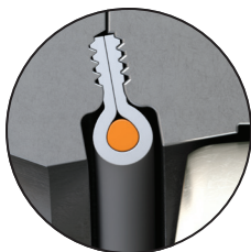
Offene Stellung. Sitz nicht komprimiert.
