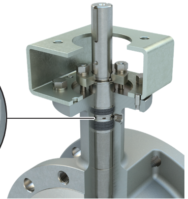
Bague D'étanchéité Solide
