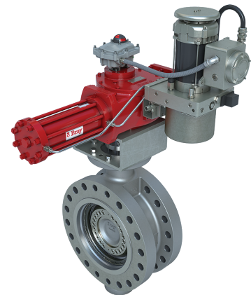
Tri Lok®-Cx montrée avec l'actionneur de la Série 98EH avec un groupe électrohydraulique.
