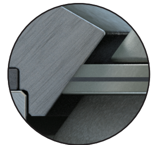
Assise Complète Lorsqu'elle est en place, la bague d'étanchéité est comprimée dans son siège sous l'effet du couple de serrage.
