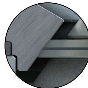
Plně uzavřená poloha V uzavřené poloze je těsnicí kroužek radiálně stlačen do sedla prostřednictvím zatížení kroužek radiálně stlačen do sedla prostřednictvím zatížení krouticím momentem.
