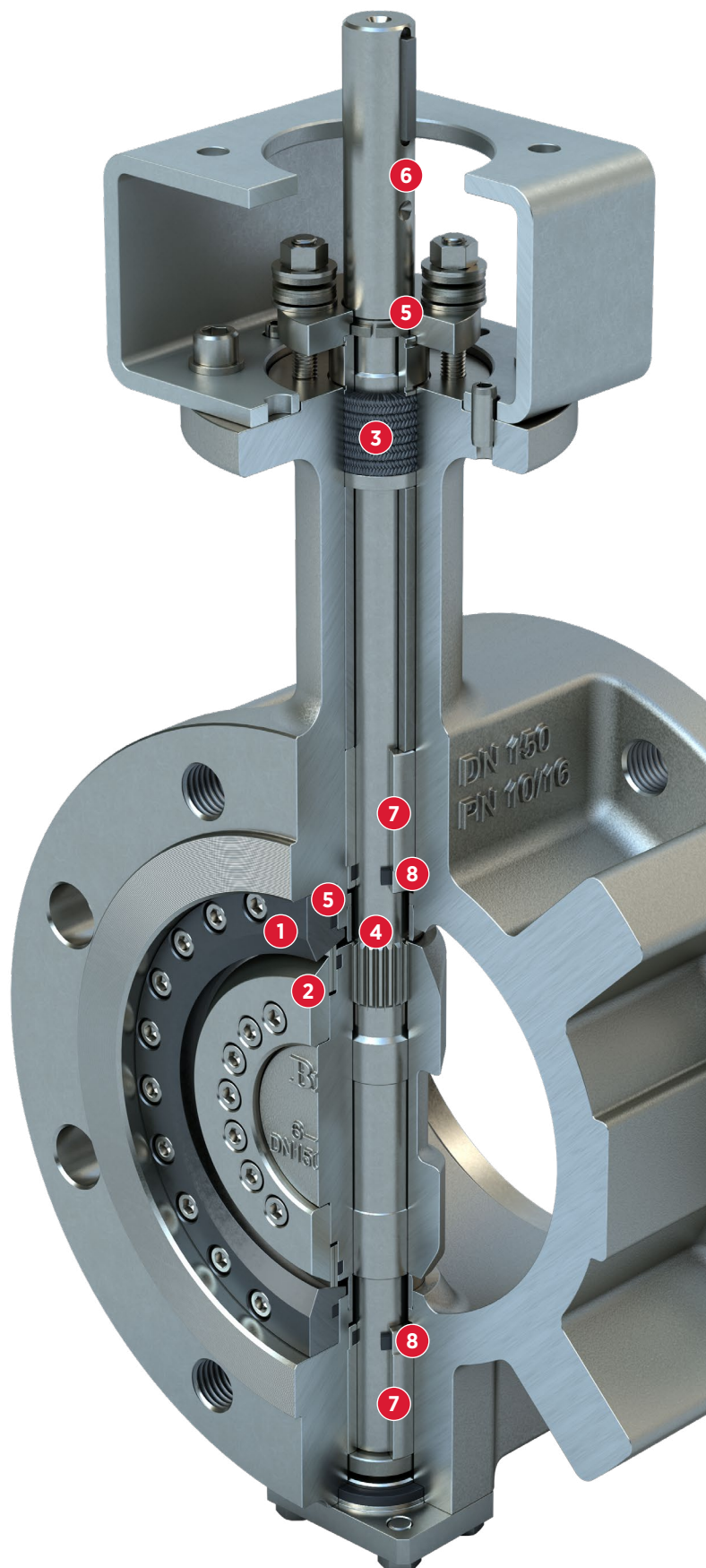
Mechanická zádržka Pro dodatečnou ochranu proti vystřelení.
