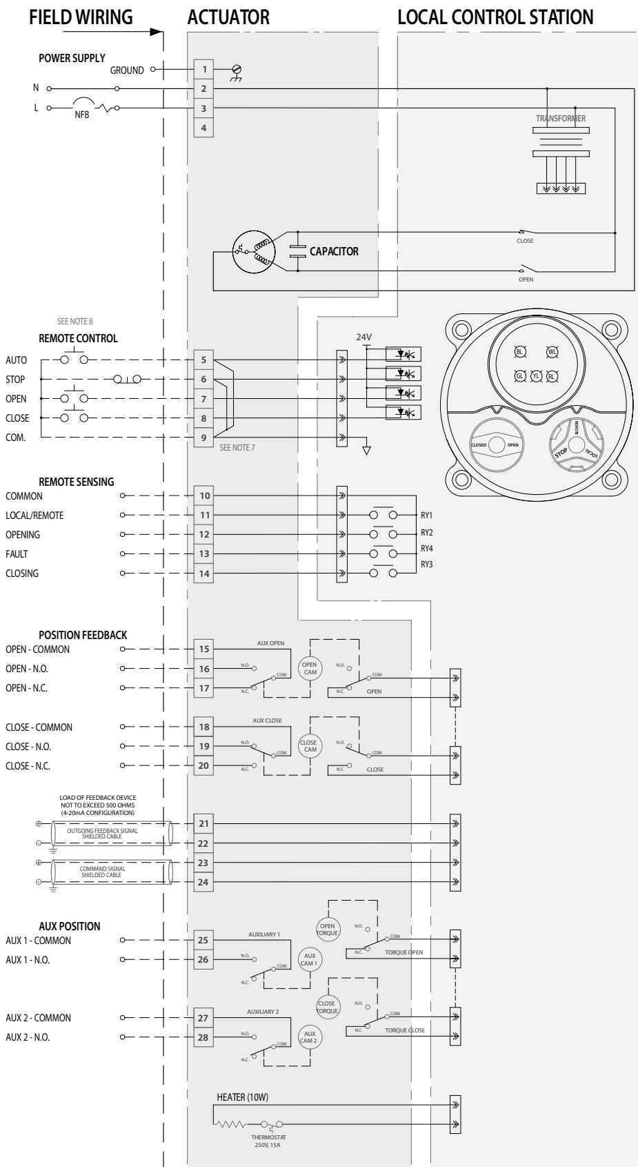
Figura 15: Ejemplo de Diagrama de Cableado para LCS Modulante
