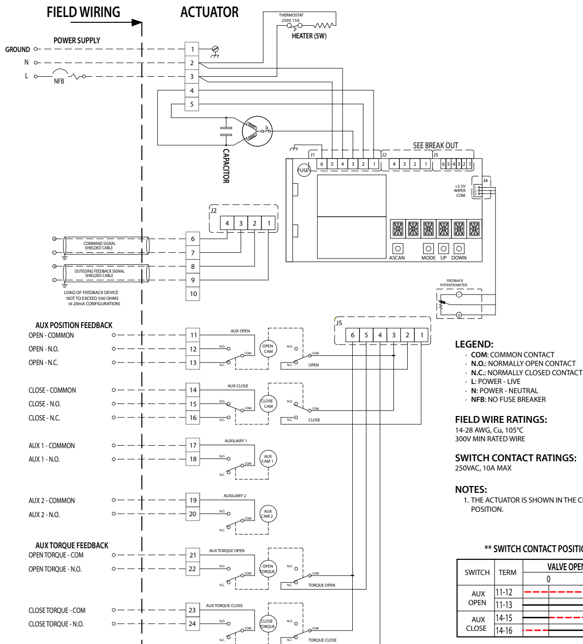
Figura 13: Ejemplo de Diagrama de Cableado: WD-000677
