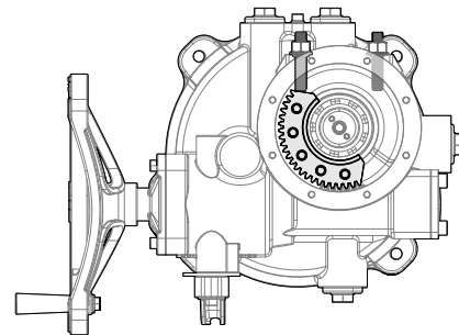
Figura 25: Tuerca y perno del tope de recorrido para CERRADO .
