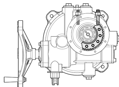
Figura 26: Caja de engranajes CERRADO .
