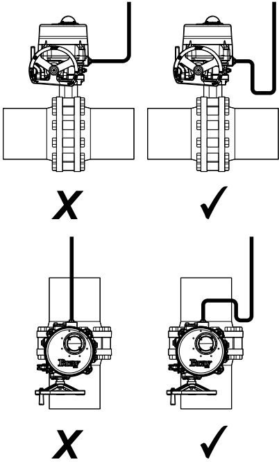
Figura 21: Enrutamiento adecuado del conducto.
