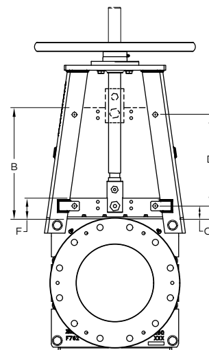
Figura 13: Ajuste de carrera
