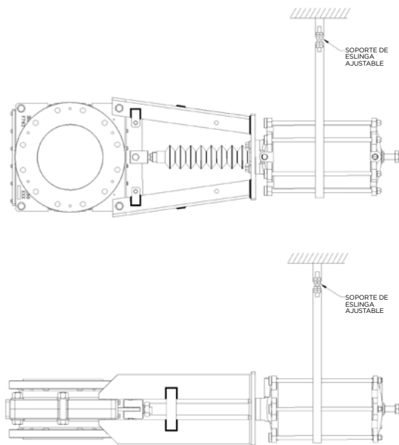
Figura 4: Válvula con Actuador
