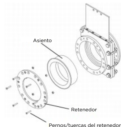
Figura 6: Conjunto de Reemplazo del Asiento
