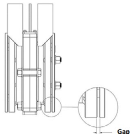
Figura 7: Brida del Retenedor y Espacio de la Carcasa
