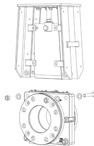
Figura 8: Desmontaje de la Compuerta
