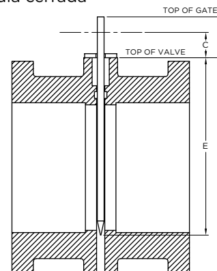
Figura 14: Ajuste de carrera, válvula cerrada
