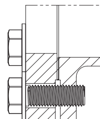
Figura 11: Parafuso da Caixa L6
