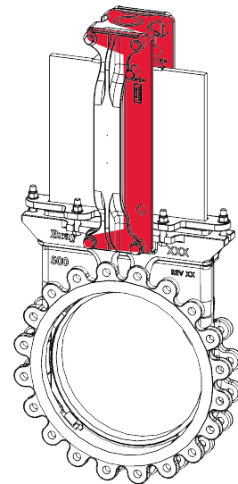
Figura 20: Pino de travamento através do suporte C.
