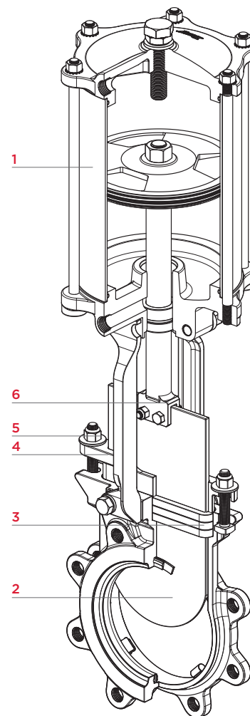
Figura 22: Vista em Corte de Válvula Operada por Cilindro
