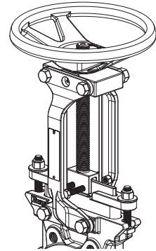
Figura 24: Incline a superestrutura.
