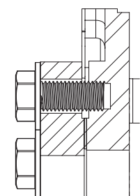
Figura 12: Parafuso Lug L7 12
