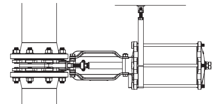
Figura 9: Suporte de instalação para uma válvula instalada na orientação horizontal (Haste horizontal e furo vertical)
