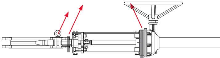
Figura 2: Válvula Guilhotina com Atuador de Engrenagem Cônica, Levantamento Horizontal
