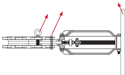
Figura 4: Válvula Guilhotina com Volante, Levantamento Horizontal
