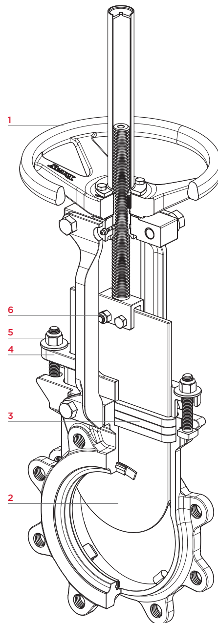
Figura 21: Vista em Corte de Válvula Manual
