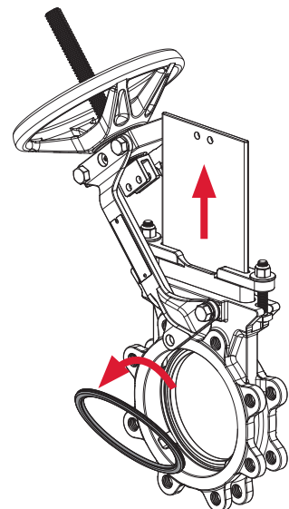
Figura 25: Levante totalmente a guilhotina e remova a sede.
