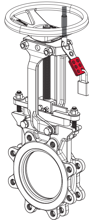
Figura 20: Pino de travamento através do suporte C.
