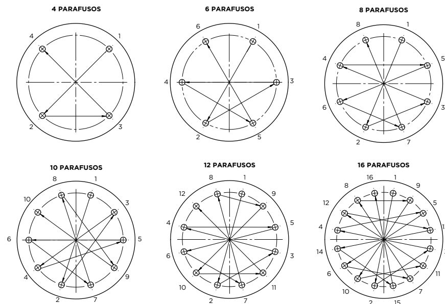
Figura 4 - Guia de Fixação de Juntas do Corpo
