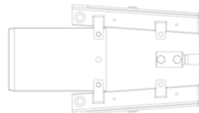
Figura 8: Remoção da Guilhotina
