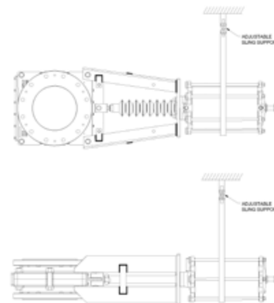
Figura 4: Válvula com Atuador
