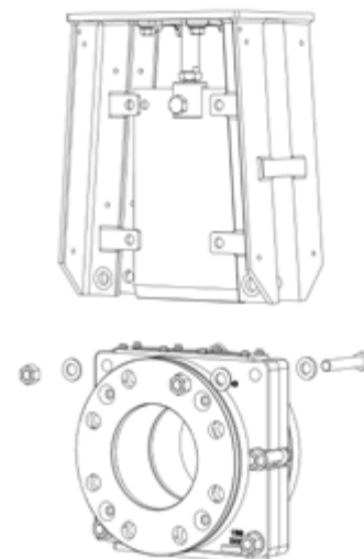
Figura 7: Desmontagem da Guilhotina
