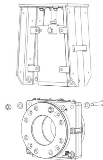
Figura 8: Desmontagem da Guilhotina
