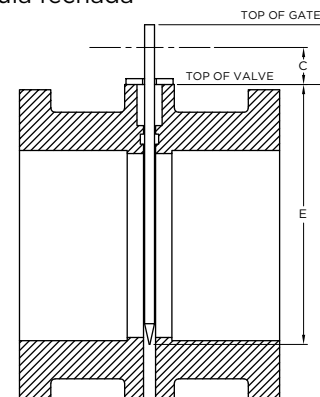
Figura 14: Ajuste do curso, válvula fechada
