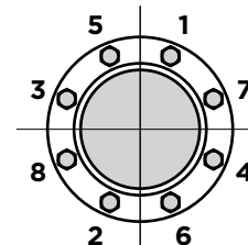
Figura 13: Padrão de Aperto dos Parafusos do Flange.
