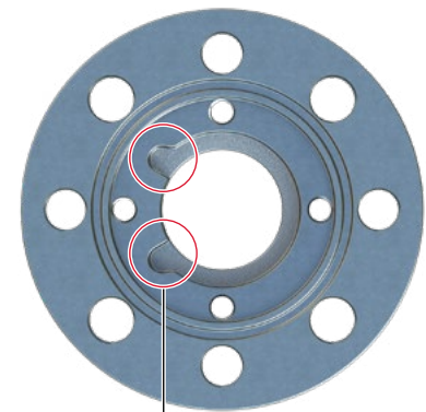
Figure 16 : Face inférieure de la retenue de presse-étoupe.
