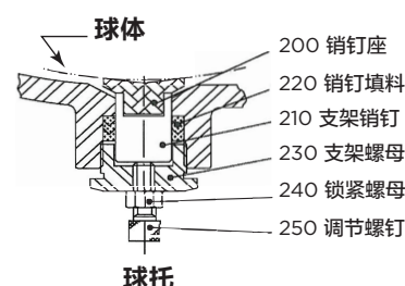
图1 - 球托结构
