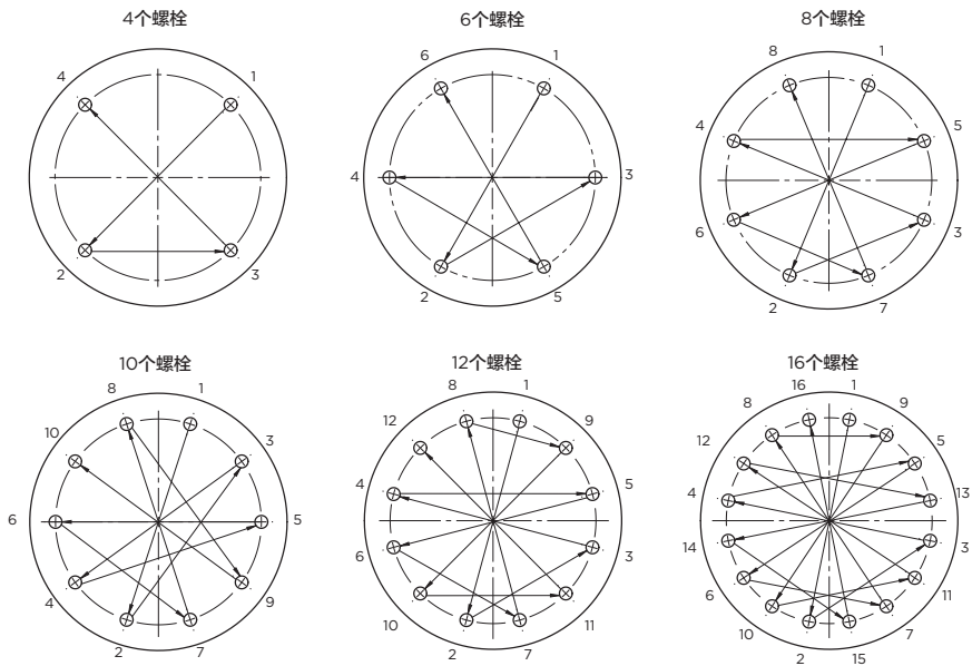
图4 - 阀体螺栓连接指南
