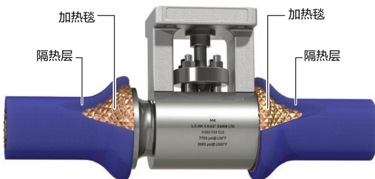
图7： 焊接后热处理（PWHT）过程的隔热保护
