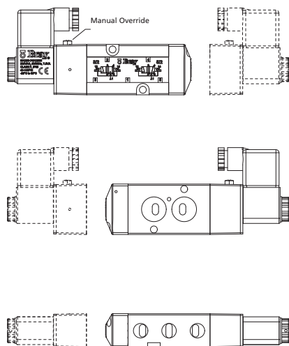
Figure 1: DIN Solenoid
