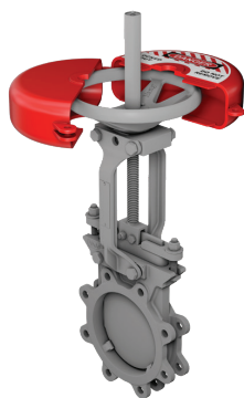
手轮锁定
